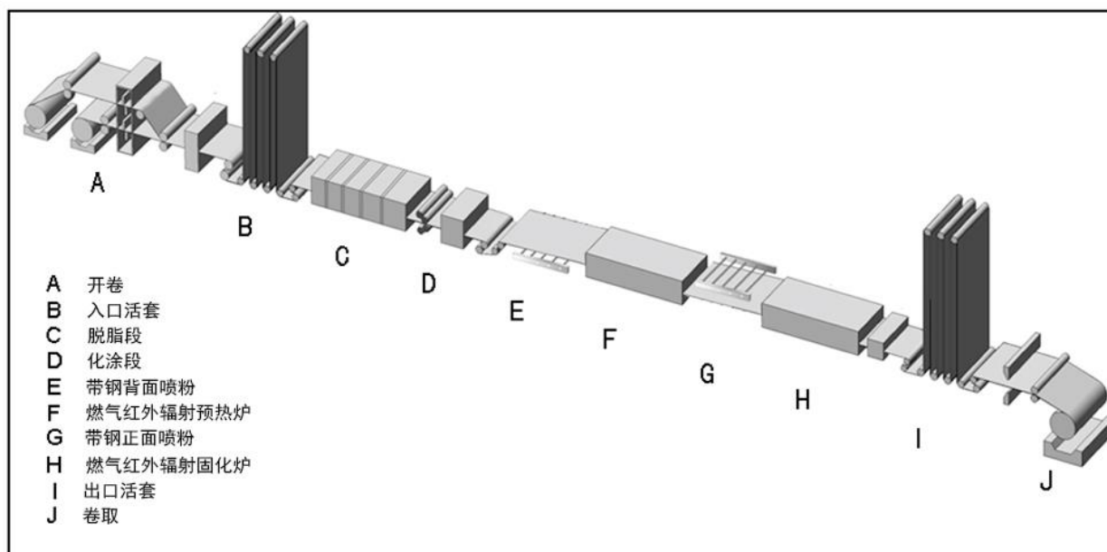
生产流程图
